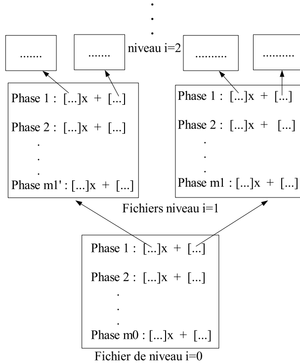
FIG. 5.1 – Croissance du nombres de fichiers pour l'exécution récursive de T
